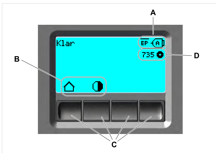
Figur 18: Elementer på kontrolpanelet på XLP 60x: A Ikoner, der informerer om interfaces konfiguration, B ikoner, ser viser tasternes konfiguration, C betjeningstaster, D visning af foliebeholdning.
