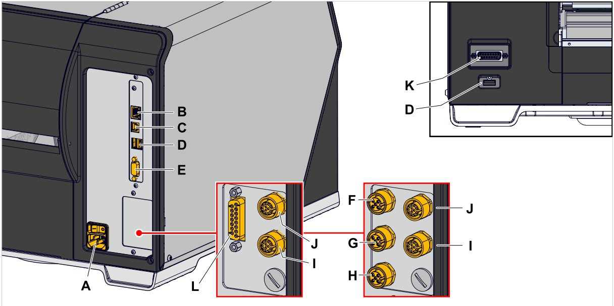
Figur 34: Tilslutninger af en XLP 60x "Peripheral", valgfrit med "BasicIO" (F-H) og "8IO" (I, J) eller med "Basic-USB" (L) og "8IO" (I, J) interfacekort.
