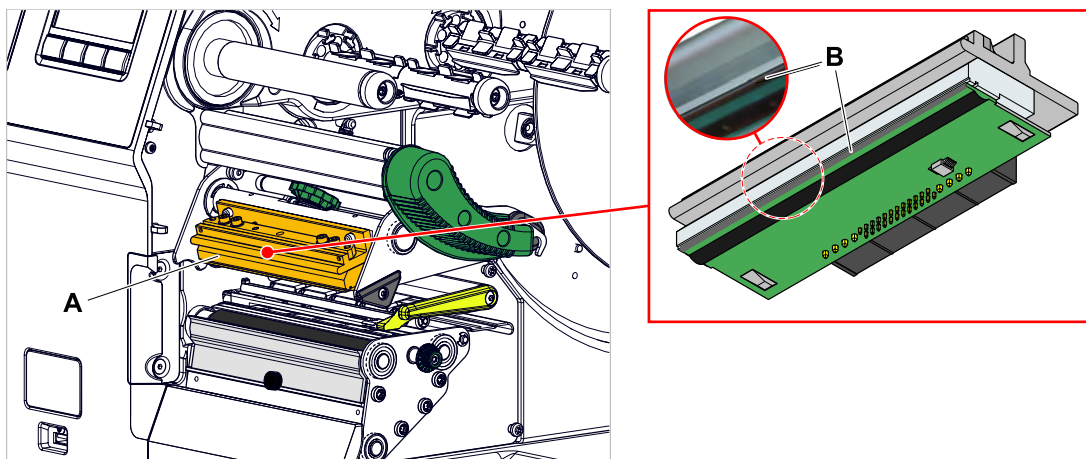
Figur 61: A: Printhead, B: Termoliste på printhead
