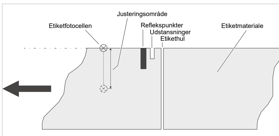
Figur 8: Etiketfotocellens justeringsområde.
