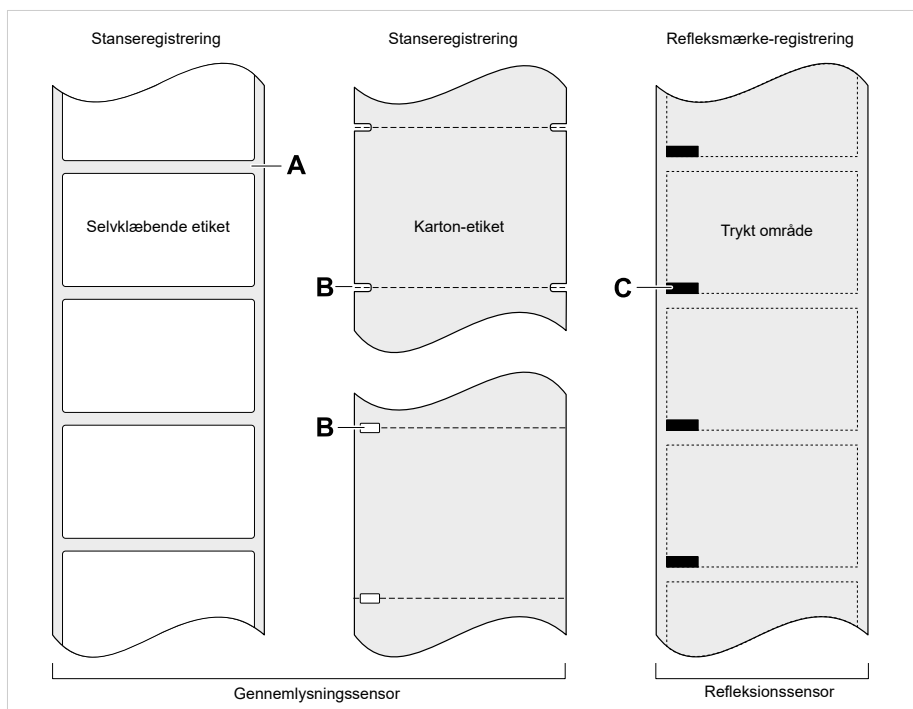
Figur 67: Forskellige typer og positioner for etiket-startmarkeringer.
